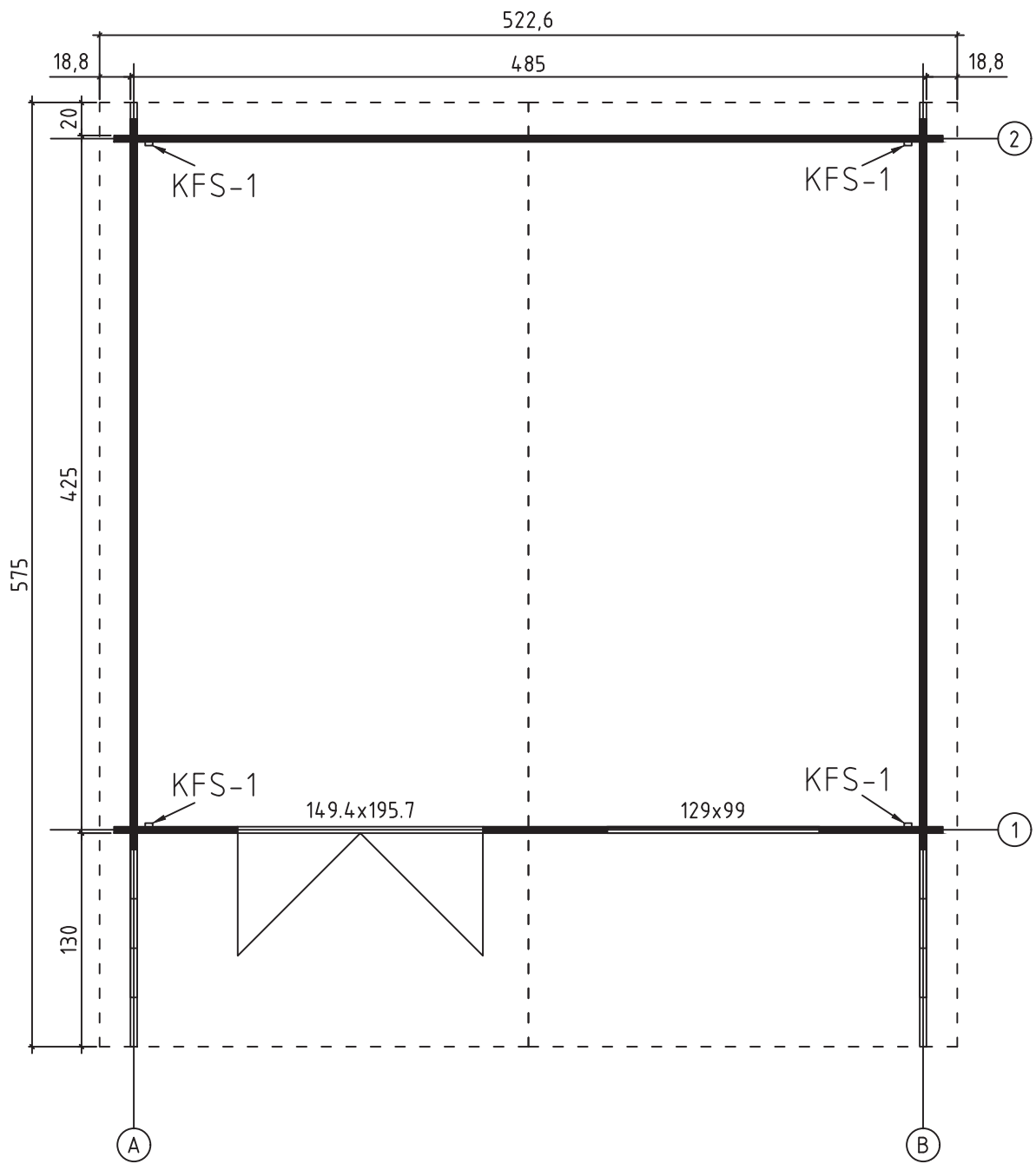
GROUNDPLAN - GRUNDPLAN - PLAN DE MASSE
